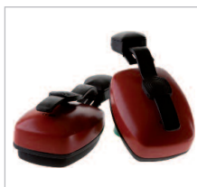
CLIPTON Ref. 82910 SNR 24 DB Protector auditivo ajustable en altura y separación. Almohadillas extra suaves para la piel. Válido para largos períodos de uso. Alta protección para trabajos en áreas ruidosas, donde deben llevarse también cascos de protección. (Ver p. 95).
